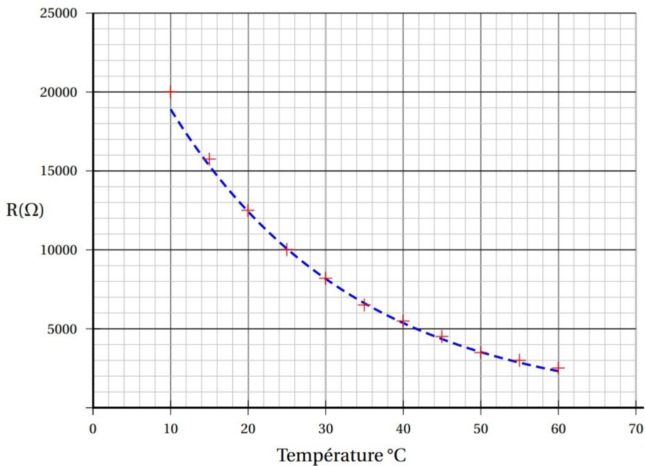
Document 2 - Résistance de la thermistance CTN en fonction de la température
