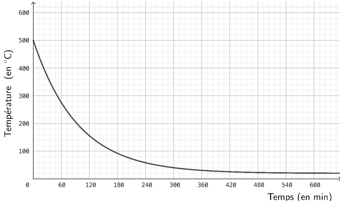
Figure 1 : évolution de la température en fonction du temps lors de la phase de refroidissement
